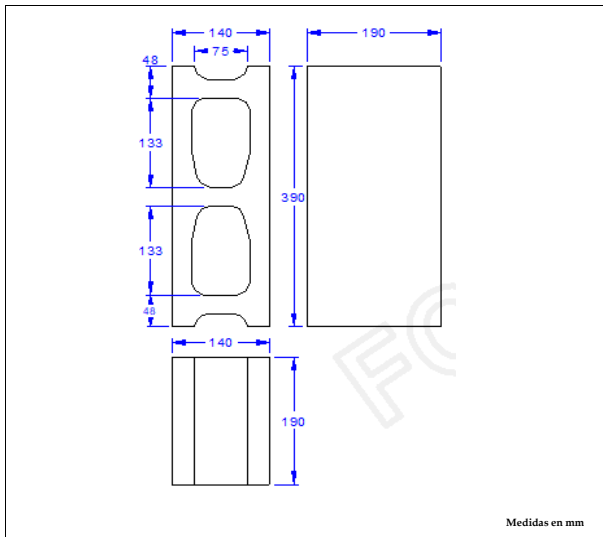
PLANO EN CORTE Y ALZADO
