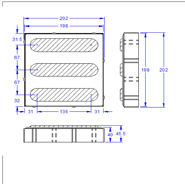
PLANO EN CORTE Y ALZADO
