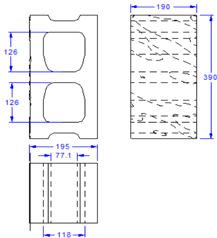
PLANO EN CORTE Y ALZADO
